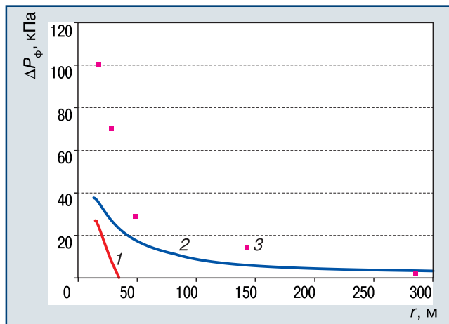
▲ Рис. 2. Изменение избыточного давления во фронте ударной волны от взрыва водородовоздушной смеси: 1 — в эксперименте; 2 — смоделированное по методике РД 03-409—01; 3 — по методике ПБ 09-540—03
