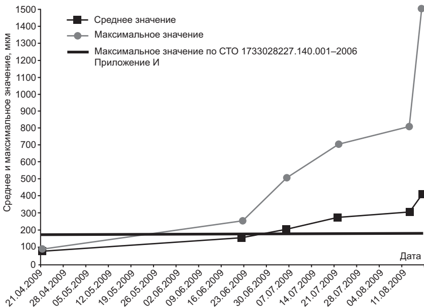
Рис. 4. Вибрация подшипника турбины второго гидроагрегата СШГЭС с момента окончания ремонта до аварии
