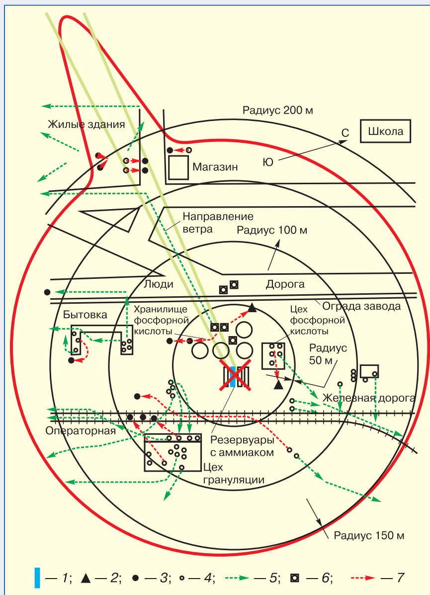
Рис. 3. Схема расположения пострадавших, в том числе погибших непосредственно на месте аварии в Потчеструме (ЮАР, 13.07.73). Красная линия — границы зоны смертельного поражения согласно расчетам по методике «Токси-3» (РД-03-26—2007), зеленая — по «Токси-2»:
